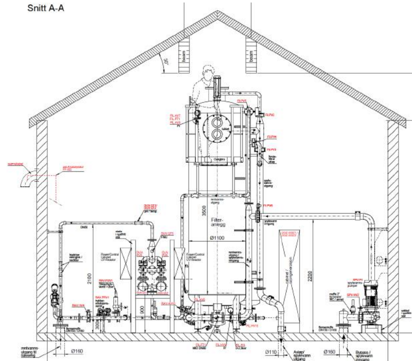
Snitt A-A
